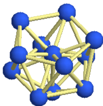
Fe12
