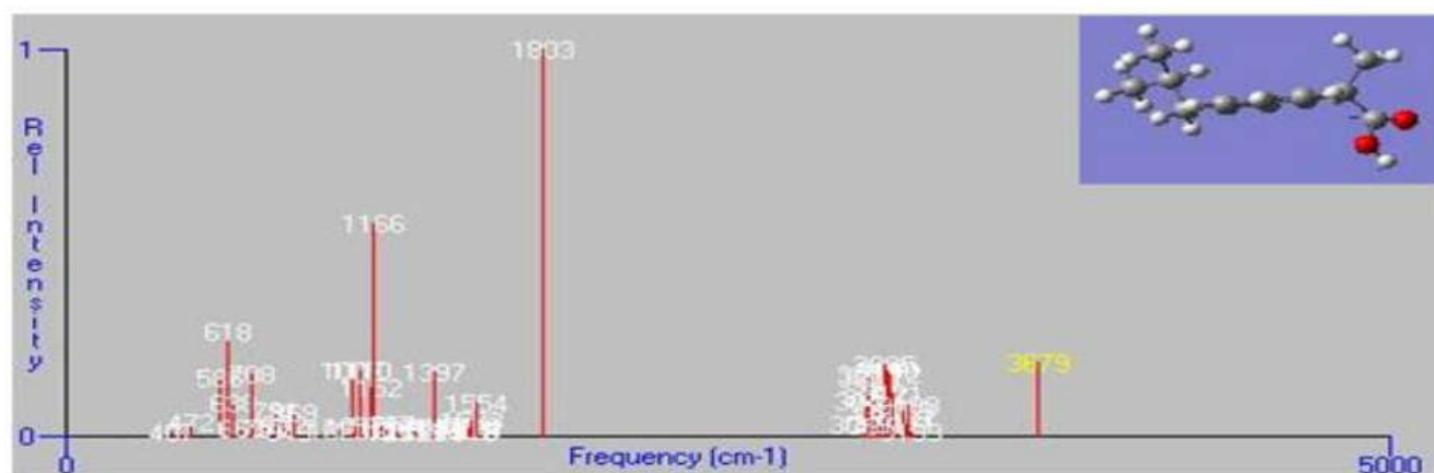
Figure 3. 28. Spectre vibrationnel IR de la molécule d'Ibuprofène dans l'ethanol obtenu avec la méthode B3LYP/6-31+G*
