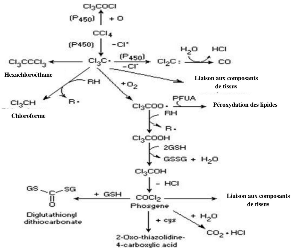
Figure 11: Biotransformation hépatique du tétrachlorure de carbone et initiation des dommages cellulaires (Recknagel et al., 1989)
