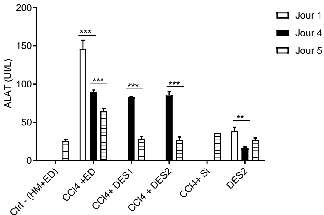
Figure 34: Effets de l'extrait de D. adscendens sur l'activité de l'ALAT un, quatre et cinq jours après administration du \text{CCl}_4
