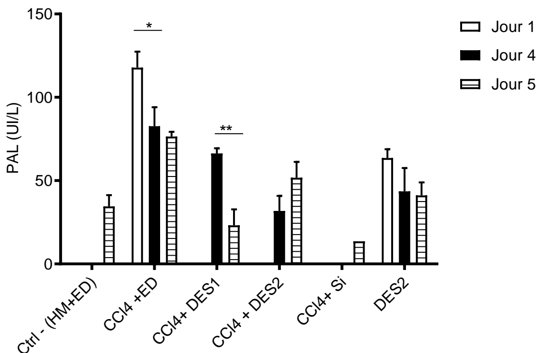
Figure 36: Effets de l'extrait de D. adscendens sur l'activité de la phosphatase alcaline (PAL) un, quatre et cinq jours après administration du CCl 4
