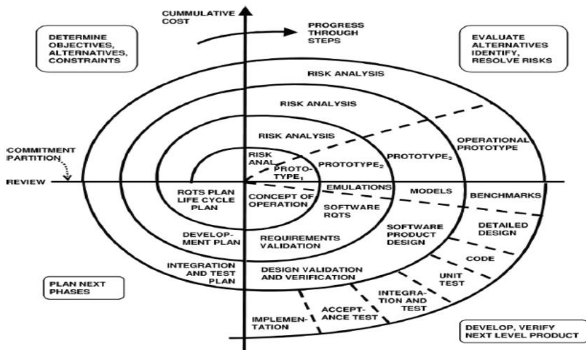
Figure 4 : Modèle en spirale
