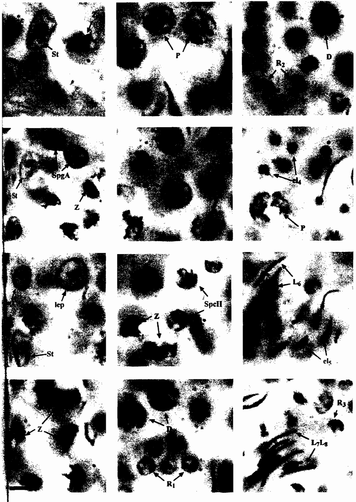
Fig. 4. Coupes de tubes séminifères de dindon adulte observés en microscopie photonique (x1575). Nomenclature issue de REVIERS (1971b) : SpgA, spermatogonie de type A ; SpgB, spermatogonie de type B ; PI, SpcI stade préleptotène ; lep, SpcI stade leptotène ; Z, SpcI stade zygotène ; P, SpcI stade pachytène ; D, SpcI stade diplotène ; SpcII, spermatocyte secondaire ; R, spermatides rondes ; el, spermatides en élévation ; L, spermatides allongées ; MB, membrane basale ; St, Sertoli ; la barre représente 10 \mu m pour toutes les photos (NOIRAULT, 1999)
