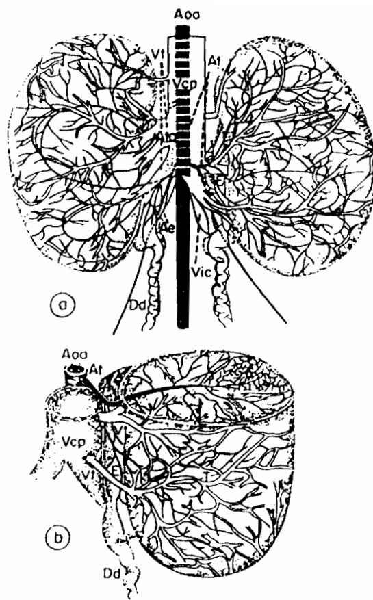
Fig. 5. Vascularisation du testicule de coq. Aoa, aorte ; At, artère testiculaire principale ; Ata, artère testiculaire accessoire ; Vt, veines testiculaires ; Ae, artère épидидymaire ; E, épидидyme ; Dd, canal déférent ; Vic, veine cave inférieure. D'après NISHIDA (1964)
