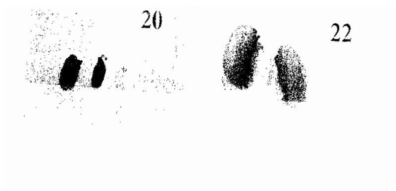
Fig. 8. Photos de testicules de pintades de T2 à 20 et 22 semaines d'âge.
