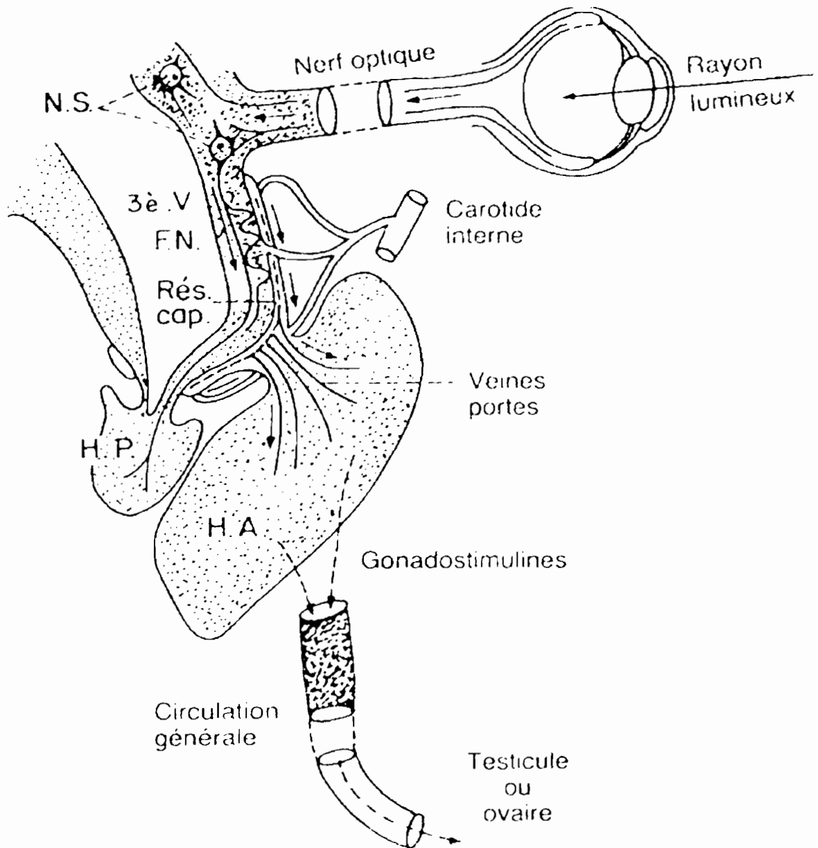
Figure 11. Schématisation du réflexe photo sexuel chez les oiseaux (d'après BENOIT et ASSENMACHER chez le canard)*
