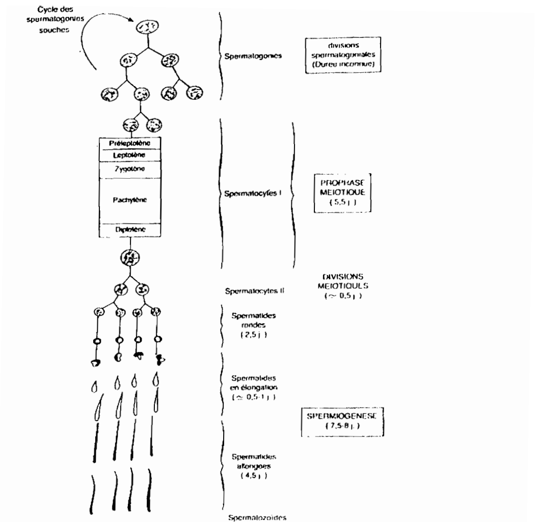
Fig. 7. Diagramme de la spermatogénèse. Le nombre et la durée des divisions spermatogoniales ne sont pas connues chez le coq. D'après de REVIERS (1988).
