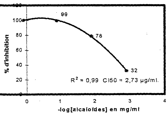
Figure 10 : Détermination des CI50 des extraits alcaloïdiques de Plante.
