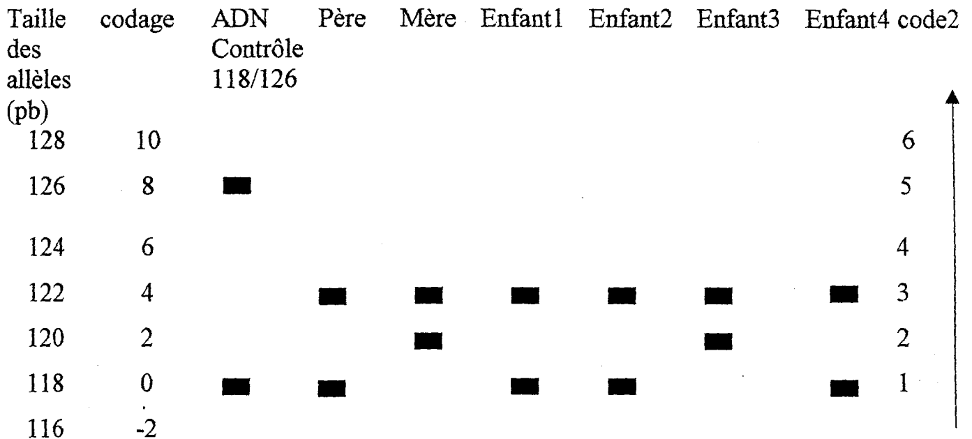
Figure 23 : Génotypes obtenus avec le marqueur D5S399.
