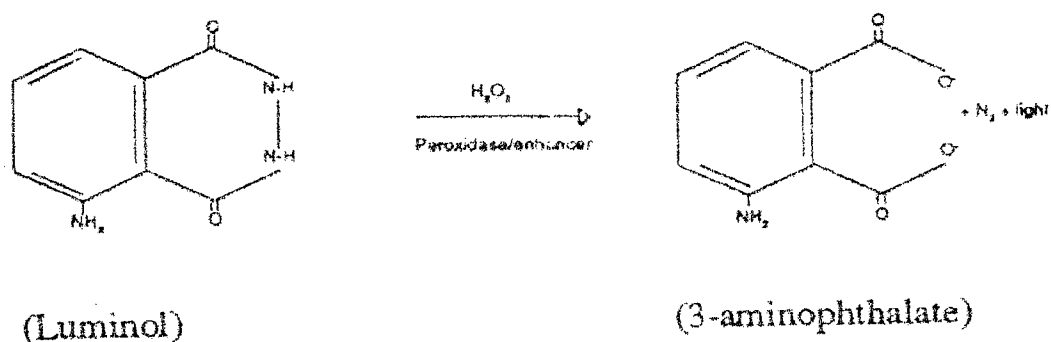
Figure 8 : Réaction chimioluminescente.
