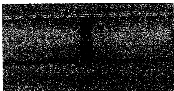
Marqueur microsatellite D5S399 amplifié.
