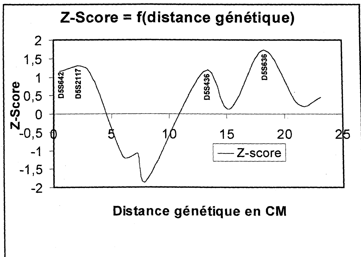
Figure 30 : Résultat de l'analyse de liaison génétique, par étude de la fréquence allélique observée dans la population étudiée.
