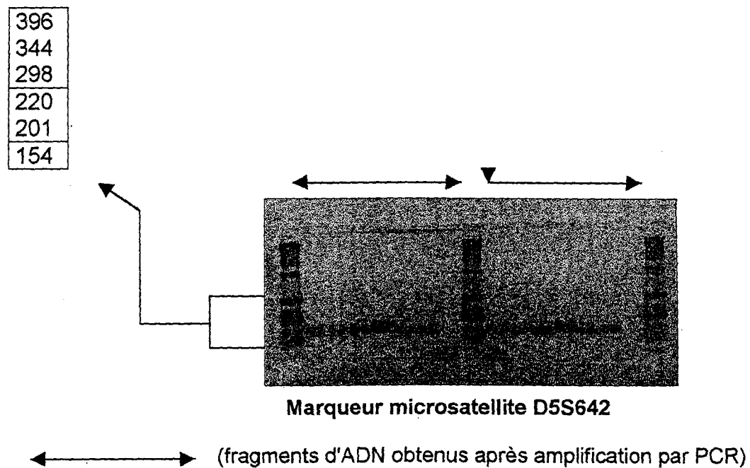
Figure 18 : Marqueur microsatellite (D5S642) amplifié par PCR.
