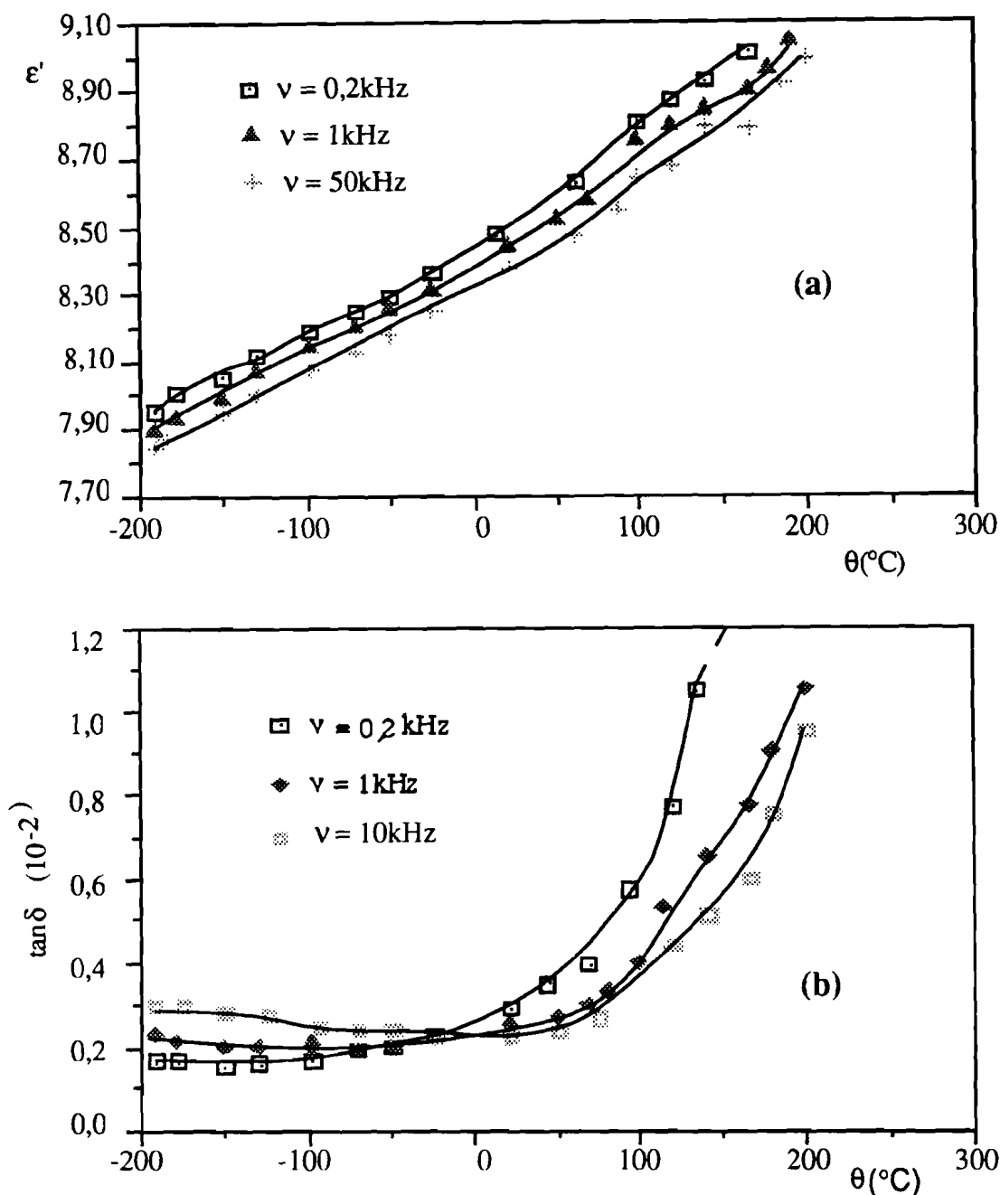
Figure 52 : Etude en fonction de la température (à différentes fréquences) d'un condensateur à base d'alumine stabilisée ( e=0,5\mu\text{m} ) : (a) variation de la constante diélectrique, (b) variation des pertes diélectriques.
