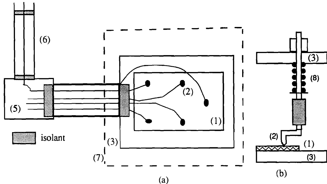
Figure 40 : Cellule de chauffage : (a) schéma d'ensemble (vue de dessus), (b) détail d'un contact électrique (coupe verticale) ; Légende : (1) échantillon, (2) contact électrique, (3) blindage de la cellule, (4) tube blindé, (5) boîte de raccordement, (6) tube coaxial, (7) étuve, (8) ressort.
