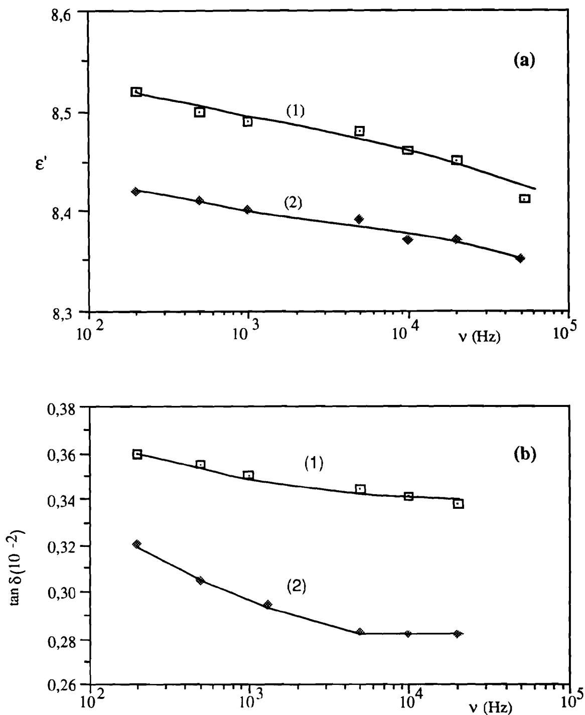
Figure 49 : Variations de \epsilon' (a) et \tan \delta (b) en fonction de la fréquence (mesurées à 20 °C) pour de l'alumine déposée à 20 °C (1) et à 250 °C (2). Les condensateurs d'étude ont une épaisseur voisine de 0,6 \mu\text{m} et une capacité proche de 2500 pF.
