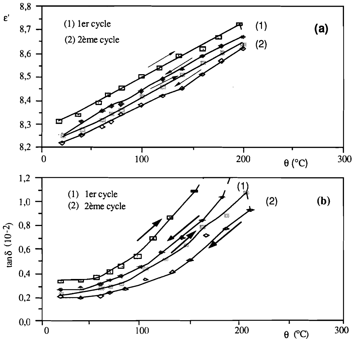
Figure 50 : Influence des traitements thermiques sur un condensateur à base d'alumine ( e=1,47 \mu\text{m} ) déposé sur un substrat refroidi (les flèches indiquent le sens de variation de la température temps de chauffage à 200 °C pour chaque cycle de 36h). Etude à 1 kHz : (a) constante diélectrique , (b) tangente de l'angle de pertes diélectriques.
