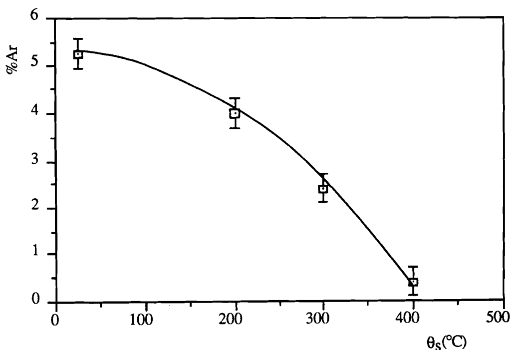
Figure 24 : Fraction molaire de l'argon dans l'alumine déposée à différentes températures du substrat (plasma Ar (98%)-O 2 (2%), pression 0,1 Pa, puissance RF 500 W).
