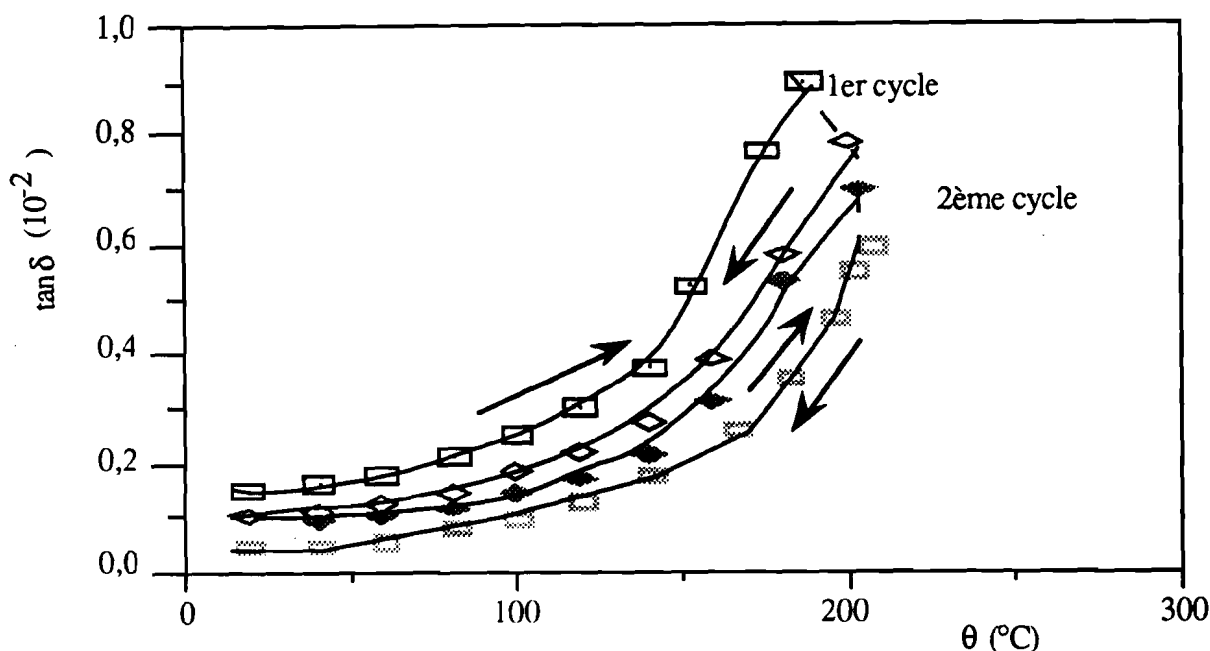
Figure 59: Variation de \tan \delta ( \nu = 1 kHz) au cours des deux premiers cycles thermiques pour un condensateur à base de \text{GeO}_2 déposé à 20^\circ\text{C} . Le temps de chauffage à 200^\circ\text{C} est de 36 h pour chaque cycle.
