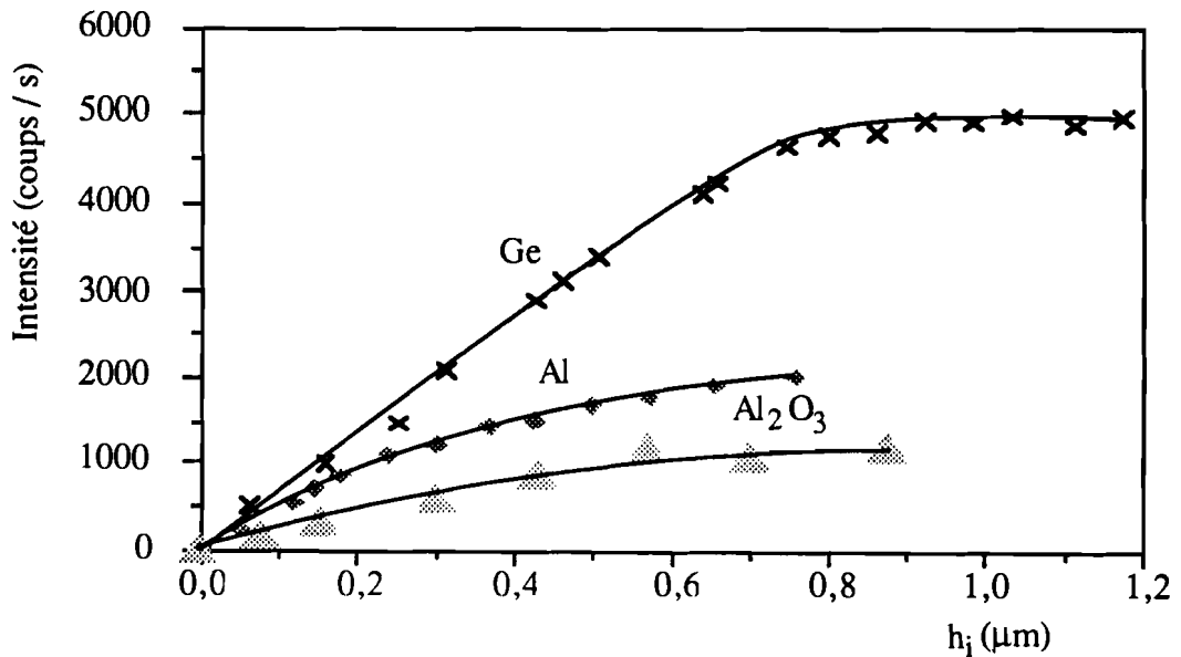
Figure 14 : Intensité mesurée par la méthode d'émission pour des couches minces de Ge, Al et \text{Al}_2\text{O}_3 ; h_i est l'épaisseur de la couche mesurée par interférométrie.
