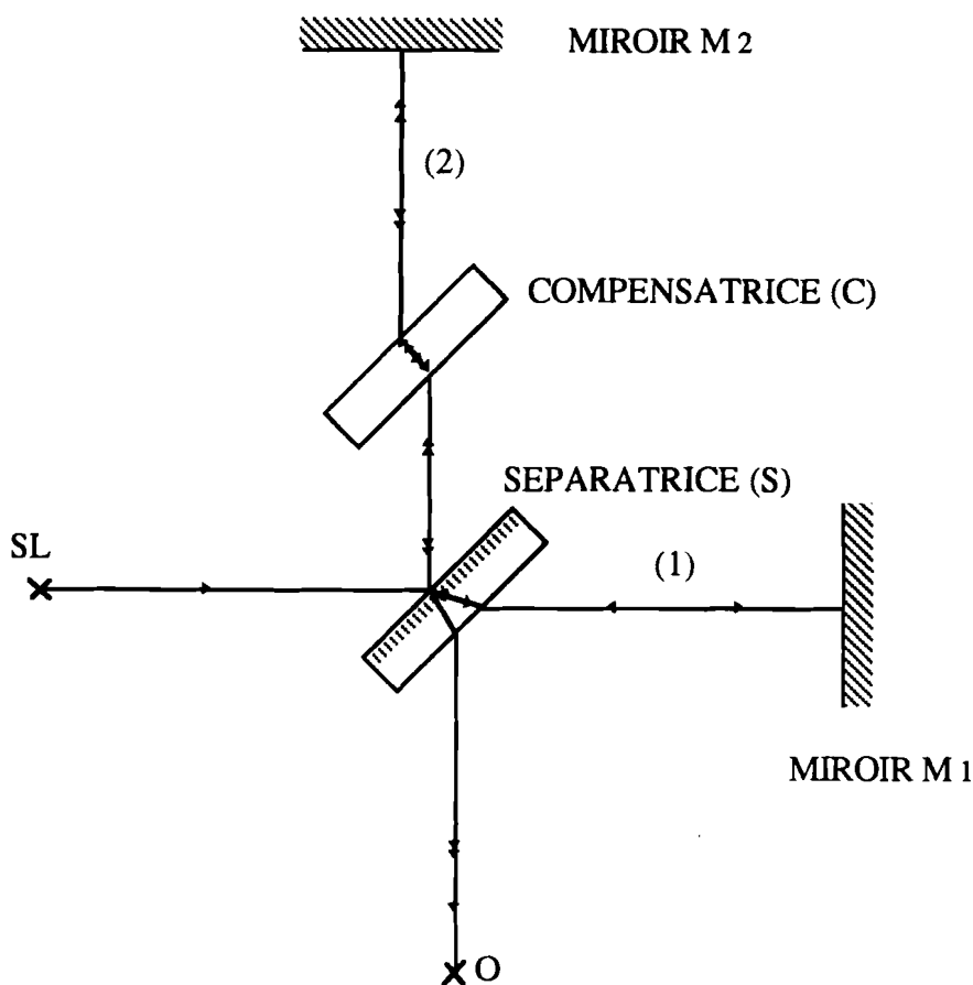
Figure 5 : Schéma de principe de l'interféromètre de Michelson.
