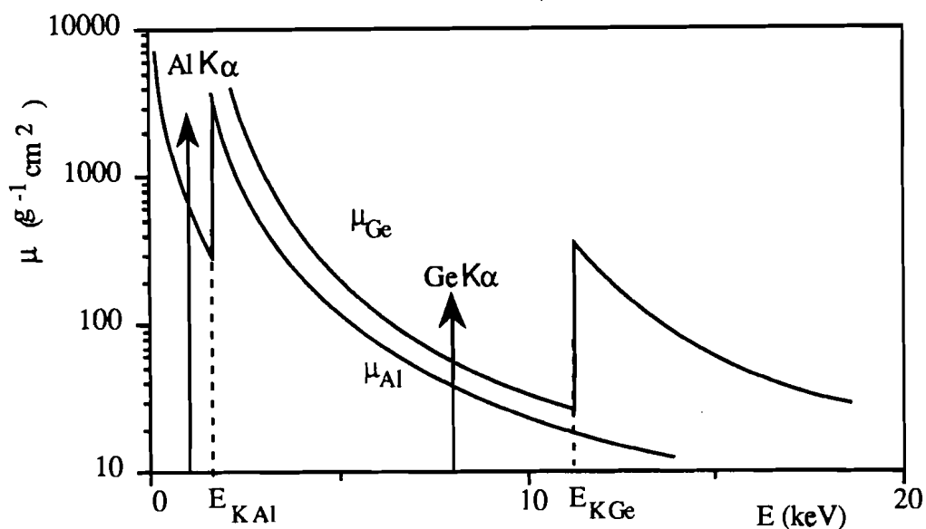
Figure 13 : Spectres d'absorption de Ge et Al comparés aux spectres d'émission GeK\alpha et AlK\alpha
