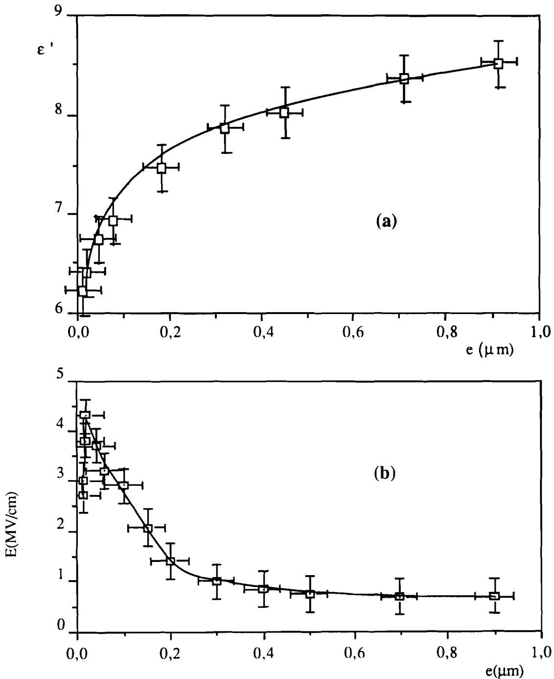
Figure 58 : Influence de l'épaisseur de la couche sur les caractéristiques de l'alumine mesurées à 20^\circ\text{C} : (a) constante diélectrique à 1 kHz, (b) champ de claquage.
