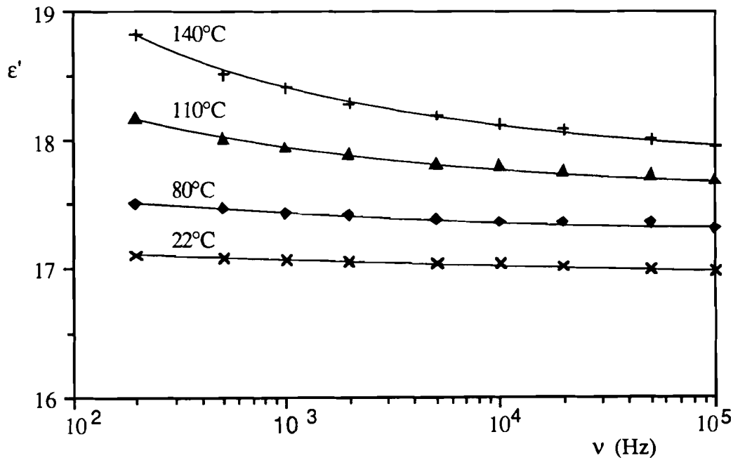
Figure 65 : Variation de la constante diélectrique de GePb_{1,4}O_{3,4} en fonction de la fréquence à différentes températures.
