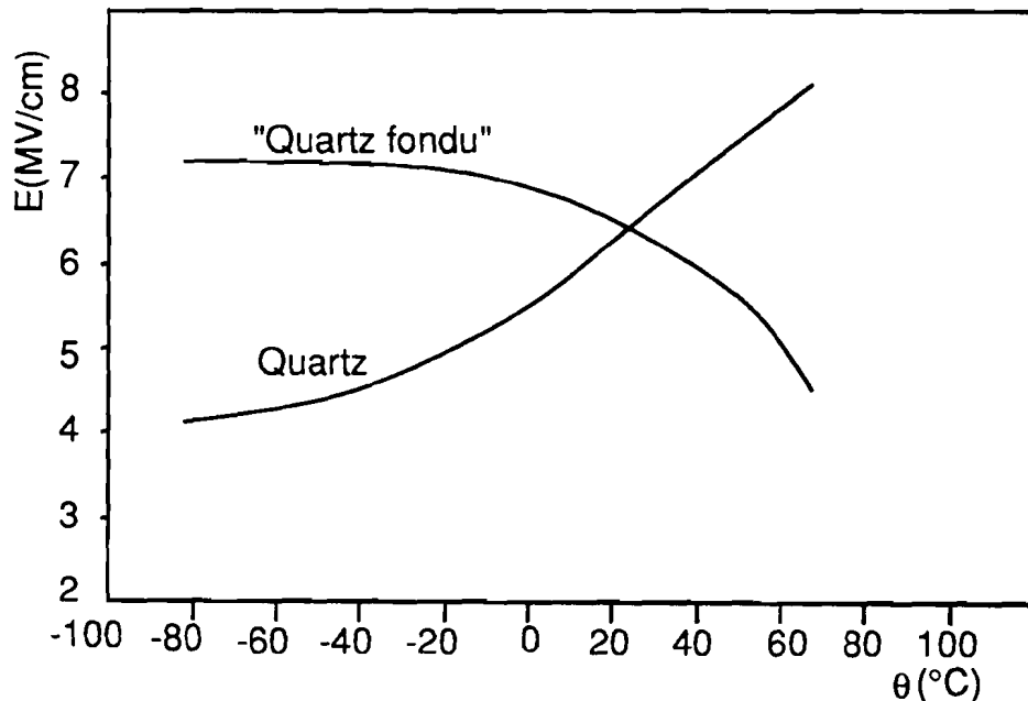
Figure 36: Comparaison du champ de claquage entre la forme cristalline (quartz) et la forme amorphe (quartz fondu) de la silice d'après Von Hippel et Maurer [88].
