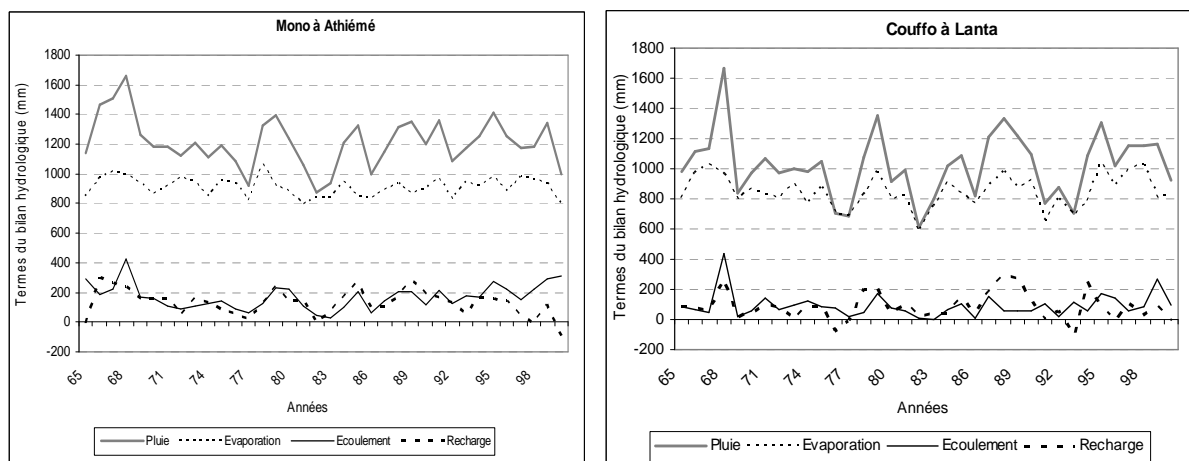
Figure 3.45 : Variation interannuelle des termes du bilan hydrologique (en mm) du bassin-versant.
