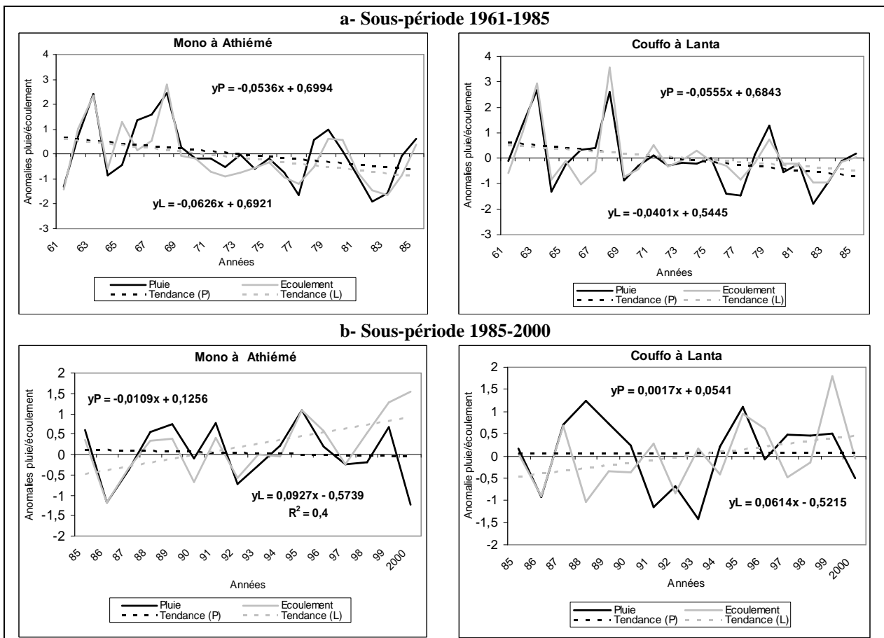
Figure 4.8 : Variation interannuelle de la pluie et de l'écoulement dans le bassin-versant du complexe Mono-Ahémé-Couffo.
