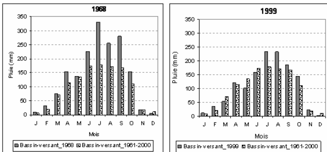
Figure 3.11 : Variation pluviométrique mensuelle (1961-2000) du bassin et des années excédentaires en amont d'Athiémi.
