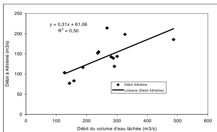
Figure 3.33 : Corrélation débit /volume d'eau lâchée dans le bassin-versant de 1988 à 2000.
