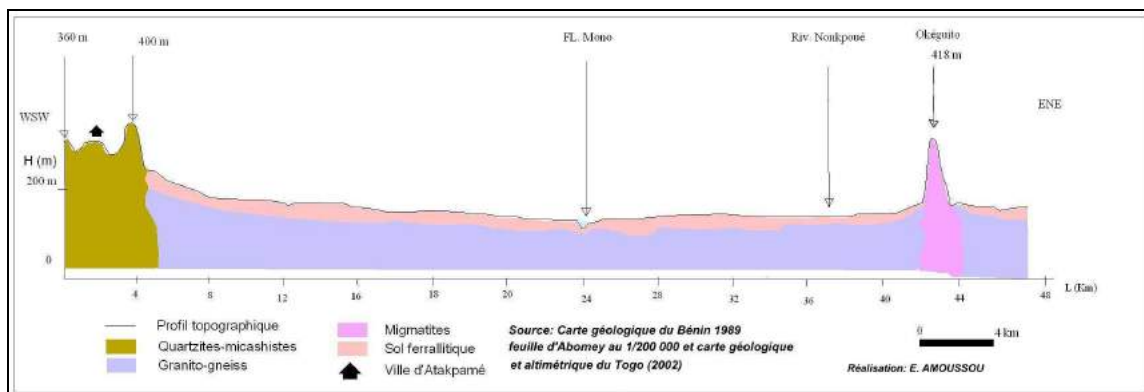
Figure 1.5 : Coupe de la pénéplaine cristalline entre le rebord montagneux (Atakpamé) et l'insertion d'Okéguito. Source : Klassou, 1996
