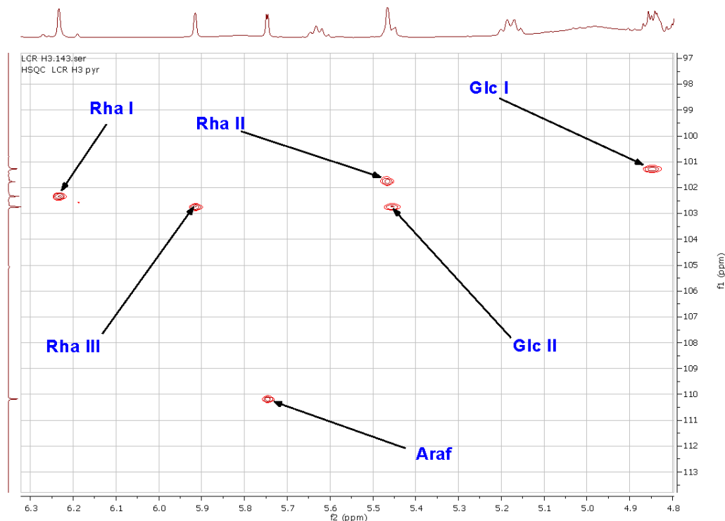
Figure 97: Spectres HSQC élargi (500 MHz, pyridine- d_5 ) montrant les signaux des anomères du composé LCR2.
