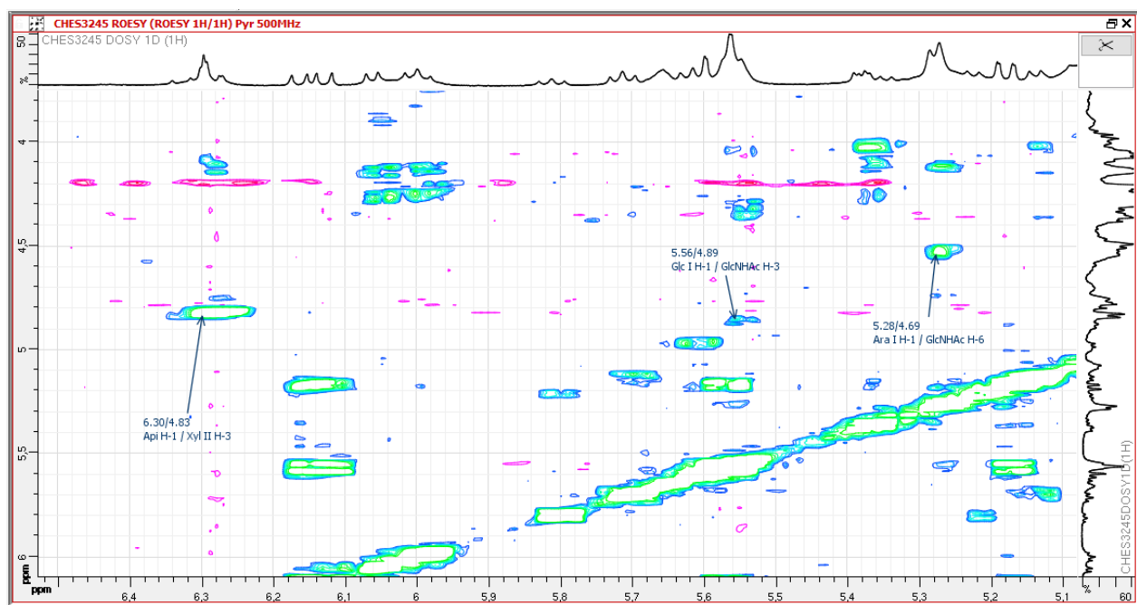
Figure 81: Spectres HMBC (a) et ROESY élargi (b) (500 MHz, pyridine- d_5 ) du composé CHEV3 montrant les points de liaison des sucres.
