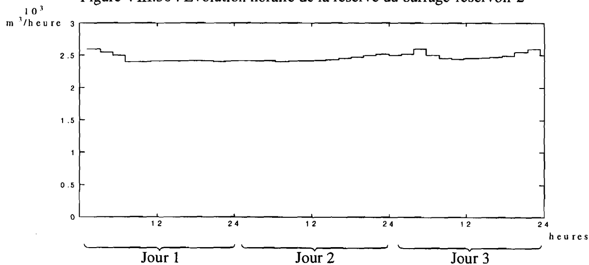
Figure VIII.30 : Evolution horaire de la réserve du barrage-réservoir 2
