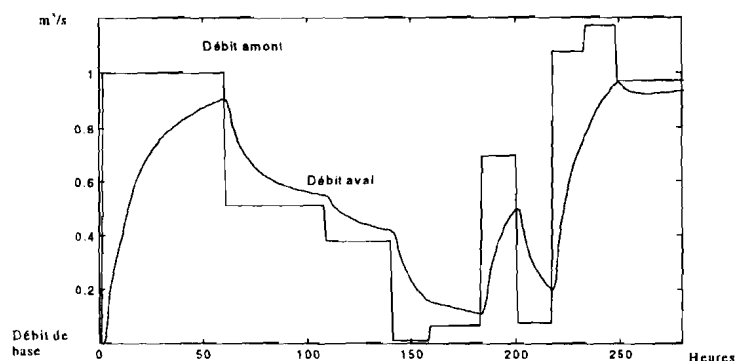
Figure V.2 : Hydrogramme d'entrée décomposé en somme d'échelons et sa réponse
