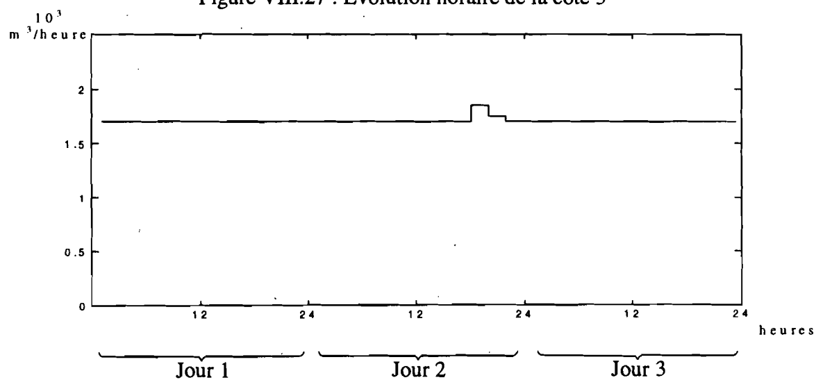
Figure VIII.28 : Evolution horaire de débit q_{34}
