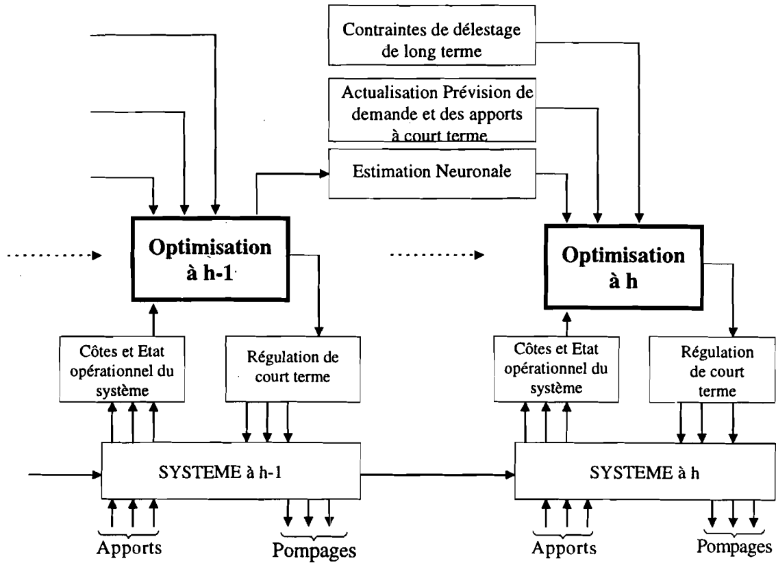
Figure VII.1 : Structure de gestion de court terme
