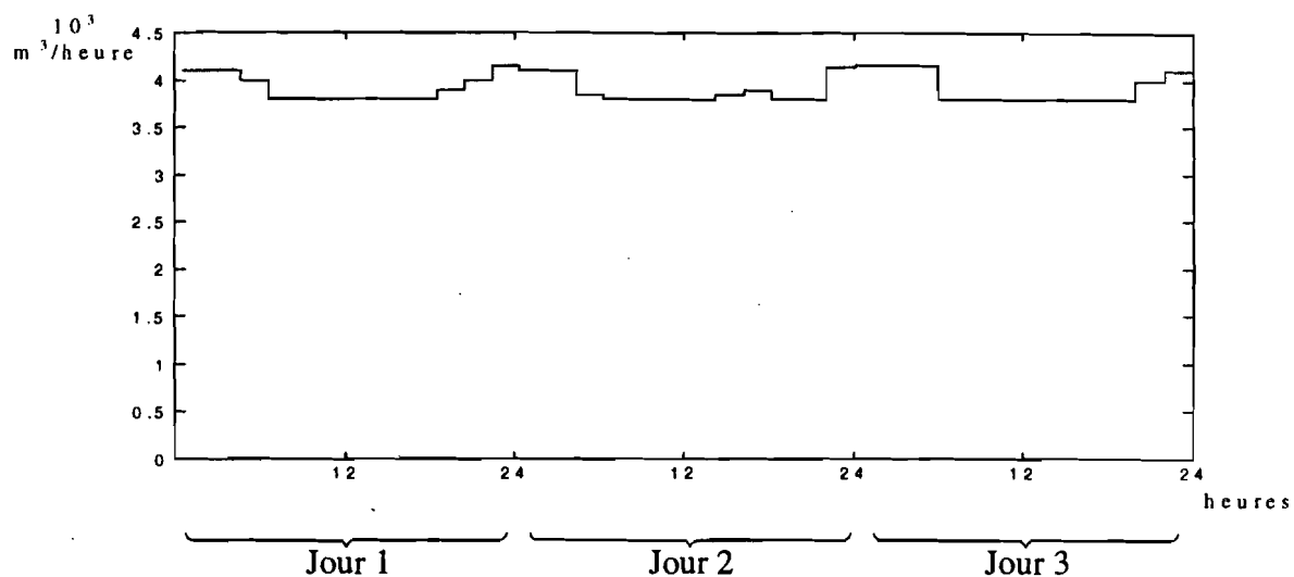
Figure VIII.26 : Evolution horaire du débit q_{13}
