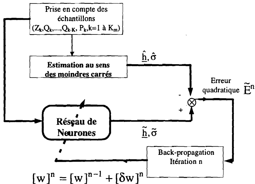
Figure V.16 : Schéma d'apprentissage retenu
