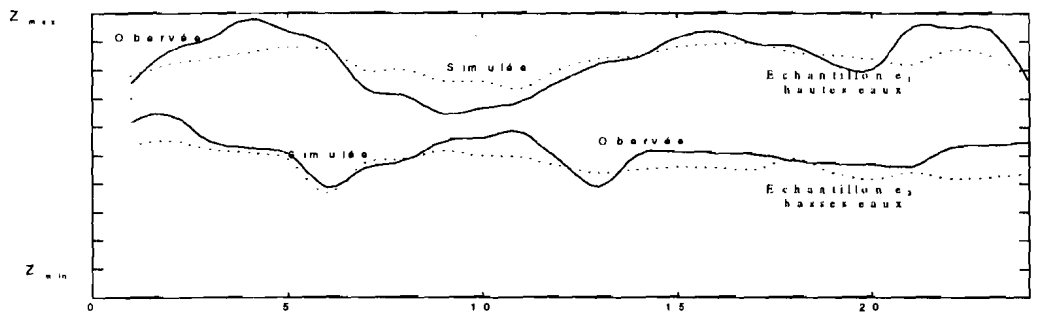
Figure V.11 : Côtes observées et simulées à l'aval d'un bief pour deux échantillons de régime de débits différents
