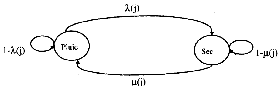
Figure III.6 : Graphe markovien des états pluviométriques
