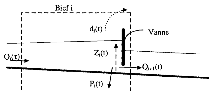
Figure V.8 : Détail d'un bief
