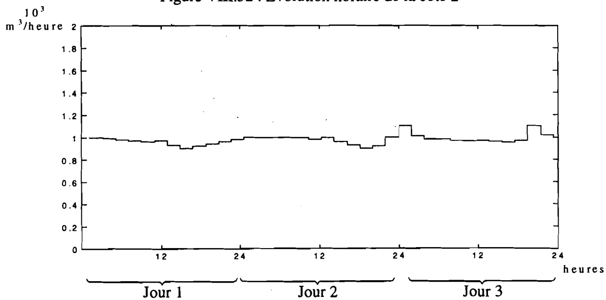
Figure VIII.33 : Evolution horaire du débit q_{23}
