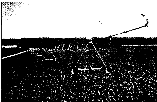
Figure A1.7 : Irrigation par aspersion [Rieul 1996]
