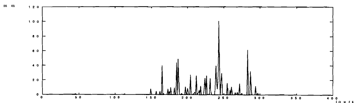
Figure III.1 : Exemple de distribution de précipitations enregistrées au Mali (Station de Bamako-aéro en 1989, source : Laboratoire d'Hydrologie de l'IRD 1 de Montpellier)
