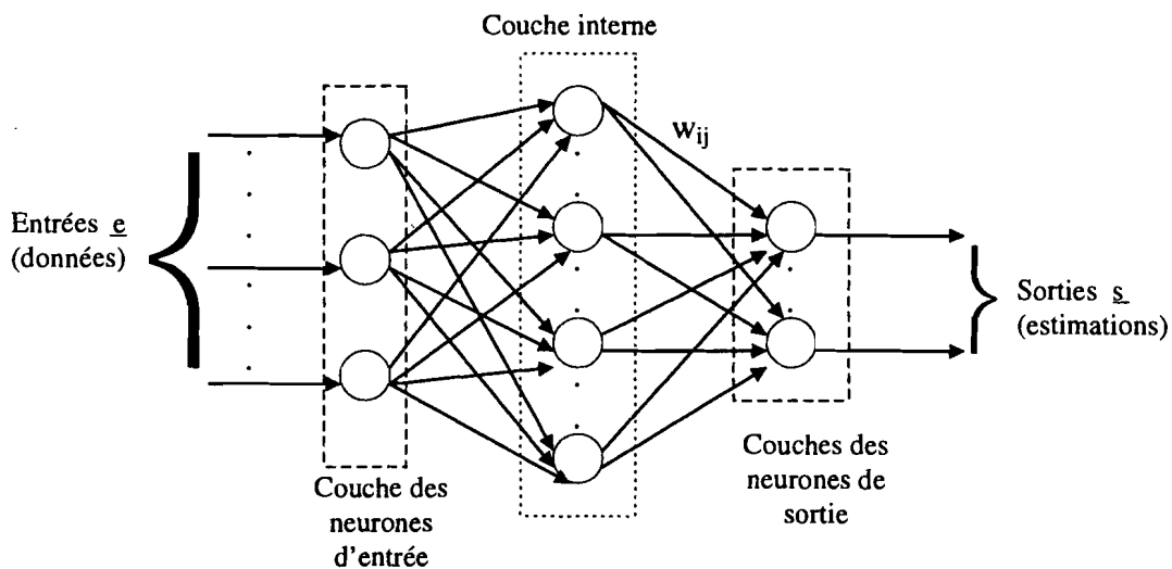
Figure A5.2 : Structure d'un réseau de neurones multicouches
